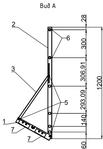
Узел крепления к кровле М1:10
