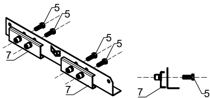
Узел крепления к кровле М1:10
