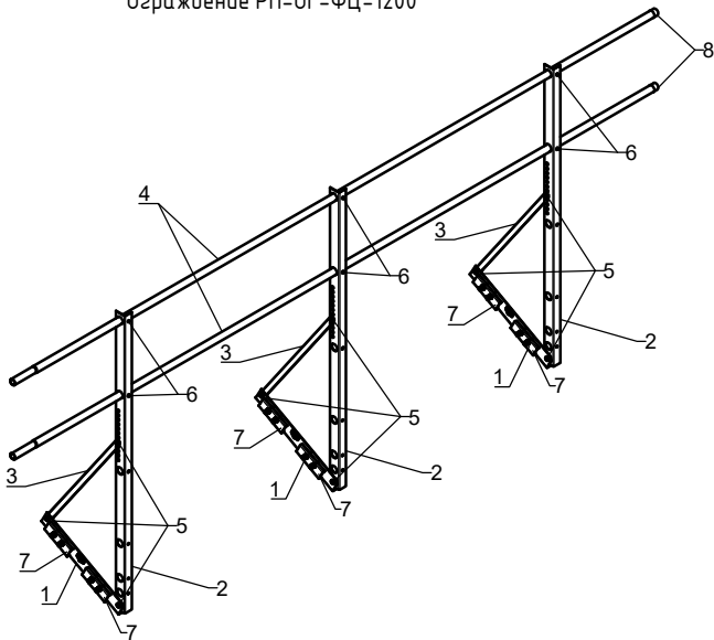
Ограждение РП-ОГ-ФЦ-1200
