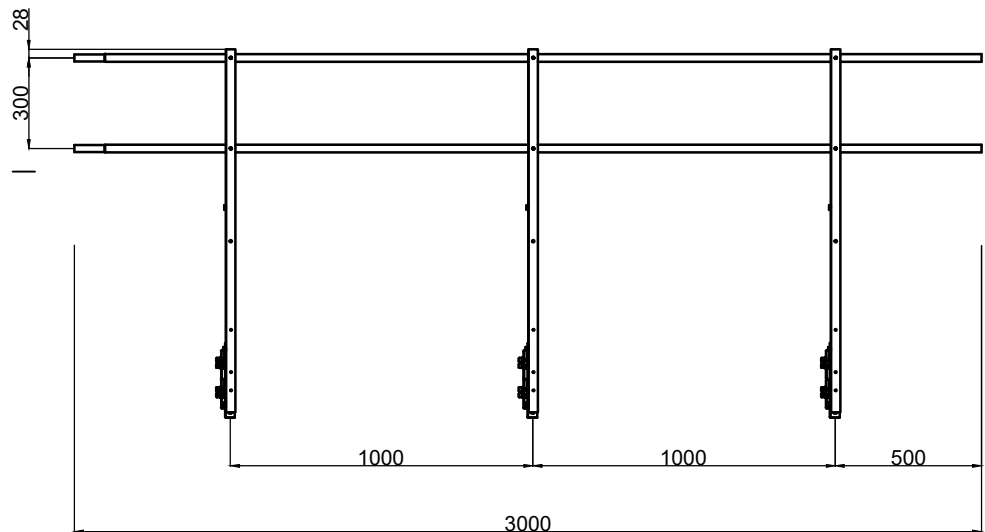
Ограждение РП-ОГ-ФЦ-1200
