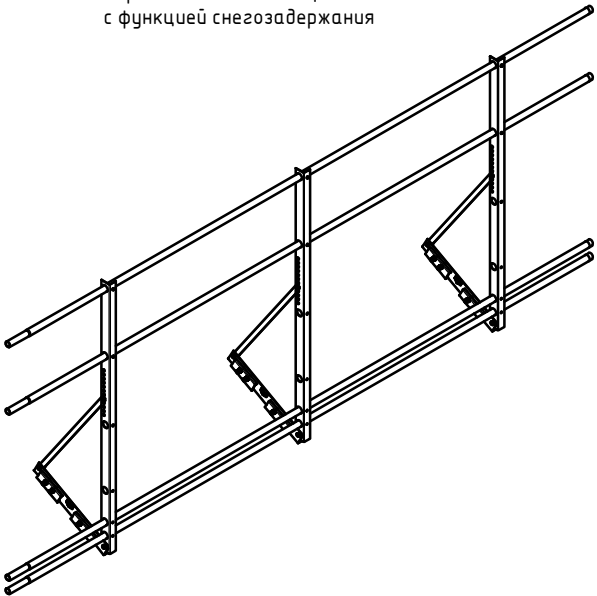
Ограждение РП-ОГ-ФЦ-1200 с функцией снегозадержания
