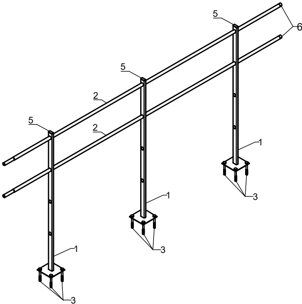
Ограждение РП-ОГ-ПР-1200
